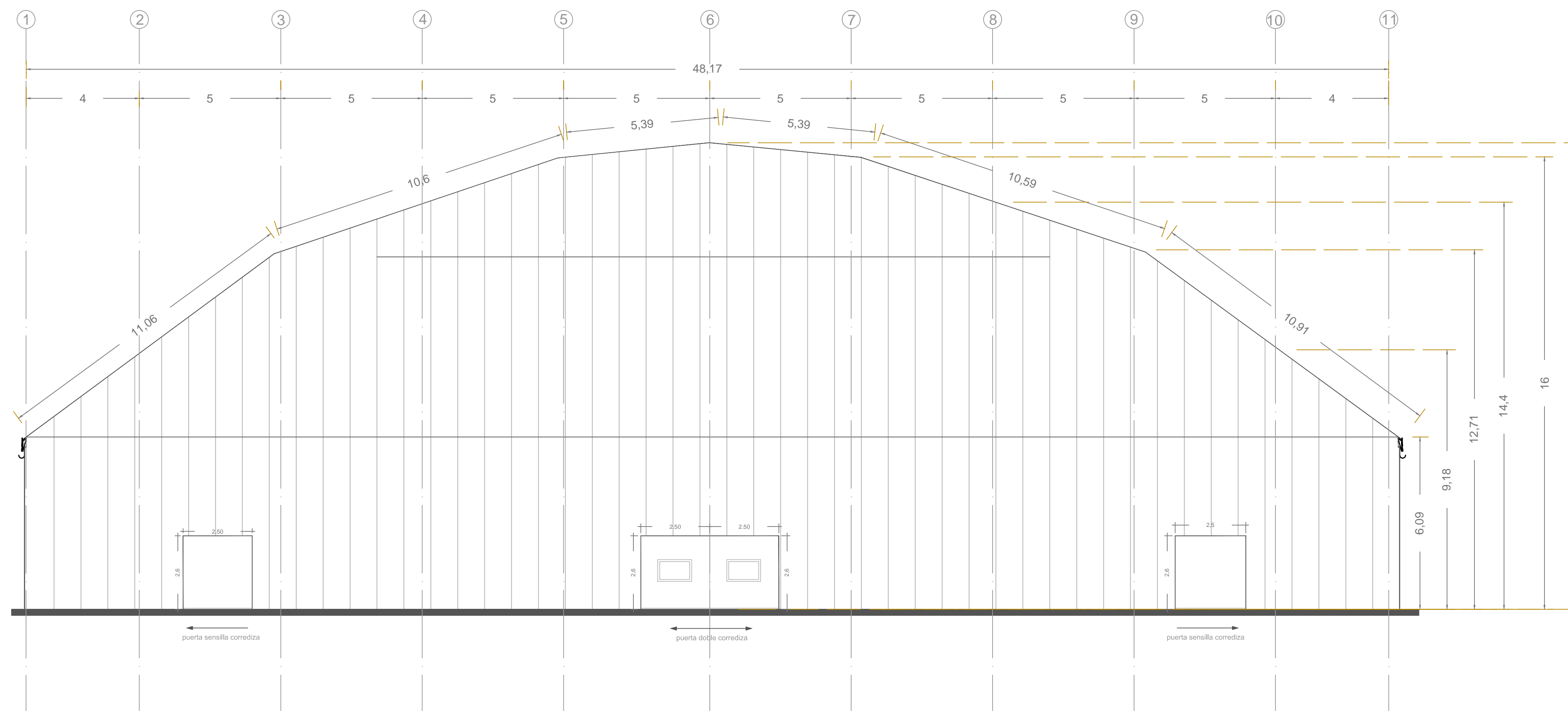
FACHADA F4/F4'
