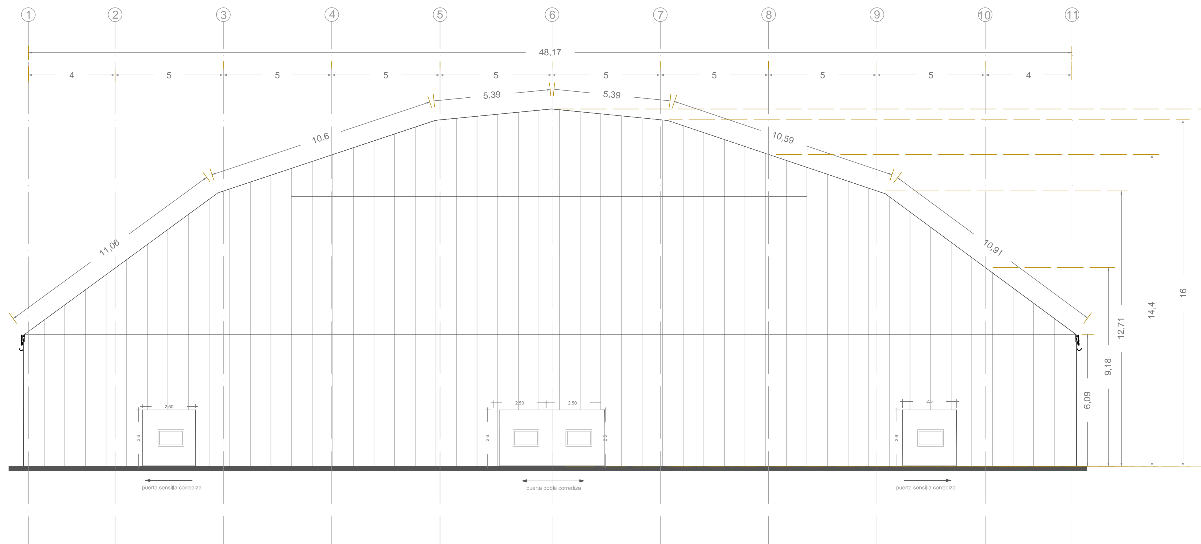
FACHADA F3/F3'
